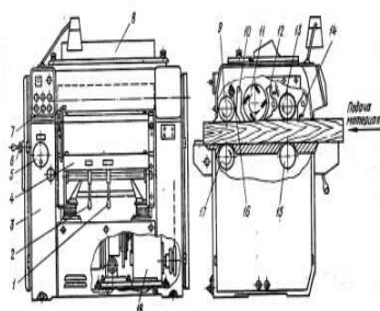
Рис. 68. Односторонний рейсмусовый станок СР6-9. 1 – рукоятка регулирования ролика; 2 – фиксатор ролика; 3 – станина; 4 – стол; 5 – механизм регулирования скорости подачи; 6 – механизм настройки стола; 7 – пружина; 8 – шариковые подшипники; 9 – задний валец; 10 – задний ролик; 11 – ножовой вал; 12 – передний ролик; 13 – передний валец; 14 – когтевая защита; 15 – опорный ролик; 16 – опорная база (фрезерный агрегат); 17 – передний валец; 18 – коробка передач.
