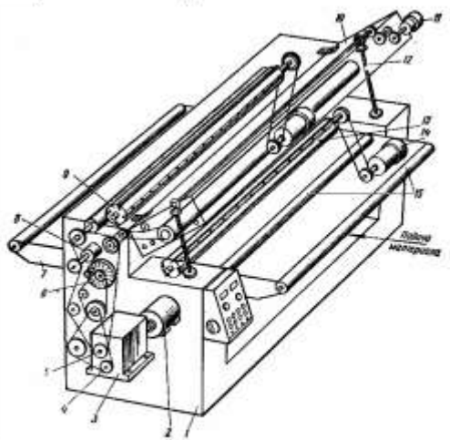
Рис. 73. Двусторонний рейсмусовый станок СРП12-2: 1 — станина, 2, 11, 14 — электродвигатели, 3 — привод с электромагнитной муфтой с возбуждением, 4, 5 — звездочки, 6 — маховик, 7 — стол, 8 — винтовой подающий валец, 9 — верхний ножевой вал, 10 — блок, 12 — винт, 13 — нижний ножевой вал, 15 — опорный ролик
