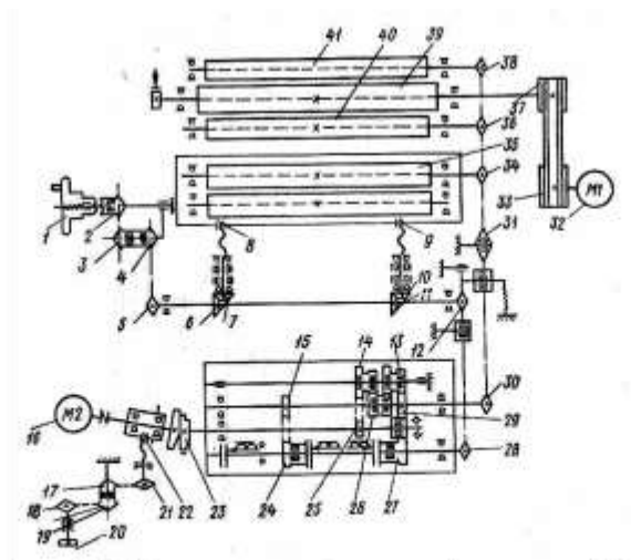
Рис. 69. Принципиальная кинематическая схема рейсмусового станка СР6-9
